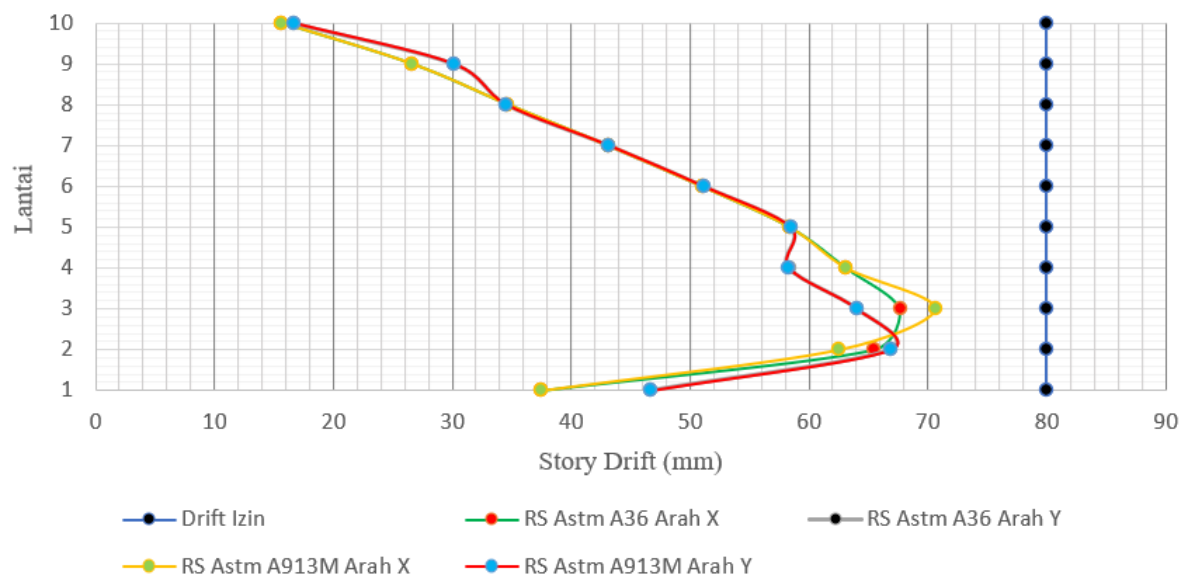
Gambar 6. Story drift respons spektrum ASTM A36 dan ASTM A913M untuk arah X dan Y
